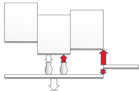
Smartbox er installeret for at undgå klemrisiko, når systemet kører op.*
